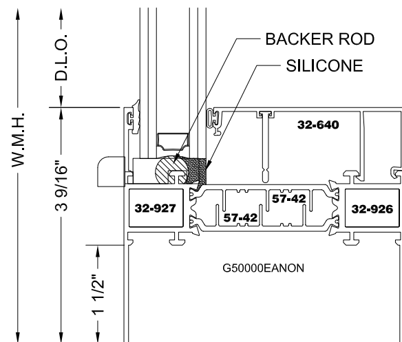
FX/PI FRAME (1-1/2\" EXT)
